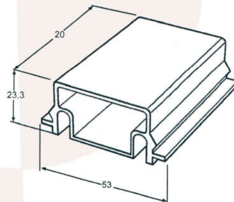
PRE 953 Presilha do forro e rodapé Alumínio Natural
