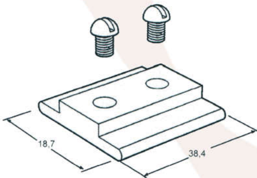
PRE 952 Presilha da coluna e travessa Alumínio Natural
