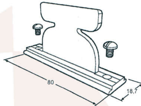
PRE 951 PV II PRE 961 PV III Presilha da coluna Alumínio Natural
