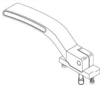
FEC 480 (Direito) FEC 481 (Esquerdo) Fecho Articulado Alumínio Preto ou Branco
