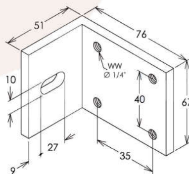
ANC 964 Ancoragem Coluna lateral Alumínio Natural (CT605)
