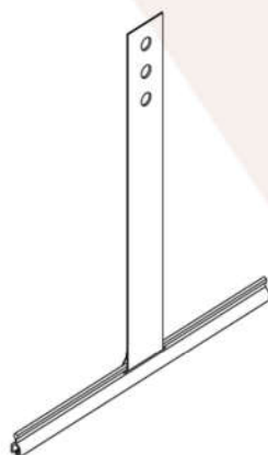
FIT 749 Mola Segurança Fixação da Esteira Alumínio / Aço mola
