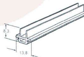
GUA 292 Guarnição do Marco EPDM
