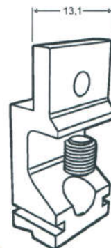
CON 360 Conexão da Travessa Alumínio Natural
