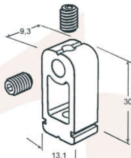
CON 320 Conexão da Travessa Alumínio Natural
