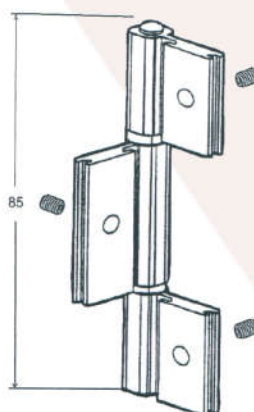
DOB 829 Fosco DOB 831 Preto/Branco Dobradiça Camarão sem Puxador
