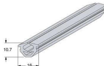
GUA 284 Guarnição Vidro 4mm EPDM
