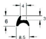
GUA 038 Baixa Guarnição Tipo Cunha EPDM
