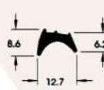
GUA 211 B Guarnição Tipo Cunha EPDM
