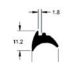
SD 813 Guarnição Tipo Cunha EPDM
