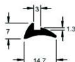
GUA 168 Guarnição Tipo Cunha EPDM
