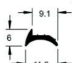
GUA 038 N Guarnição Tipo Cunha EPDM
