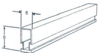
GUA 003 Guarnição de Engate L-25 EPDM
