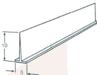
GUA 005 Guarnição Recobrimento PV EPDM
