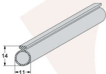
GUA 007 Guarnição da Pingadeira EPDM
