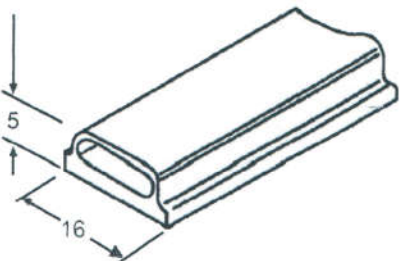
GUA 155 Guarnição Batente Jan.4FI MP EPDM
