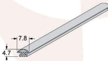
GUA 053 Guarnição Maxim-Ar EPDM
