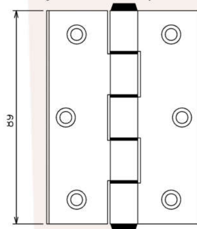
DOB 743 (Fosca) DOB 745 (Preta ou Branca) Dobradiça Alumínio Sobrepor
