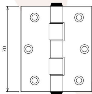
DOB 740 (Fosca) DOB 742 (Preta ou Branca) Dobradiça Alumínio Sobrepor
