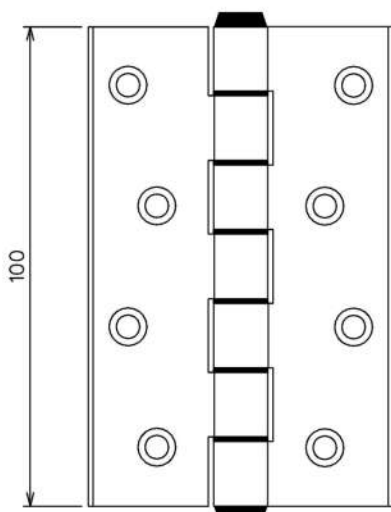
DOB 746 (Fosca) DOB 748 (Preta ou Branca) Dobradiça Alumínio Sobrepor
