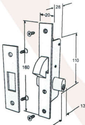
FRA 836 (Preta, Branca) FRA 845 (Cromada) Fechadura Porta de Correr
