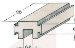
NYL 279 Calço da Folha Fixa (Porta) Nylon
