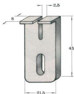
NYL 278 Guia e Trava de Segurança Nylon
