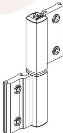
DOB 690 (Fosco) DOB 692 (Preto ou Branco) Dobradiça Tubular L-25 Alumínio
