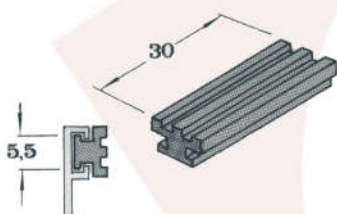
NYL 034 Guia Deslizante L-25 Nylon
