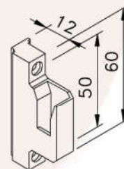
FEC 998 Contrafecho L-25 Nylon Preto
