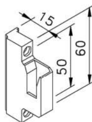
FEC 990 Contrafecho MP Nylon Preto
