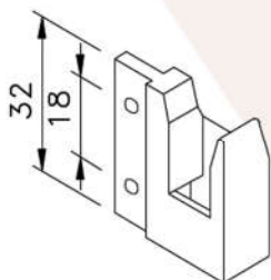
FEC 988 Contrafecho Veneziana Nylon Preto
