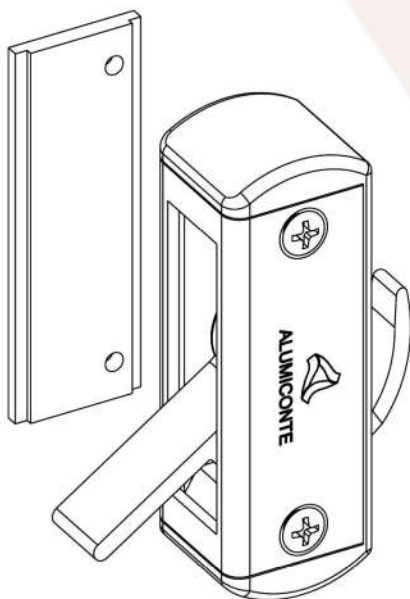
FEC 060 Fecho Caracol Linha Suprema Alumínio Preto ou Branco
