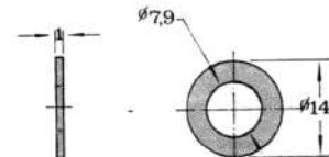
ARR 681 Arruela Pantográfica Nylon Preto
