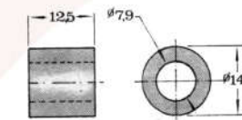
BUC 768 Buchas p/ Eixo da Tesoura Nylon Preto
