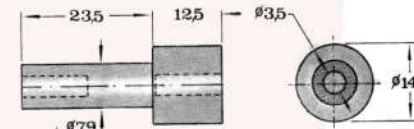
NYL 199 Eixo da Tesoura Nylon Preto
