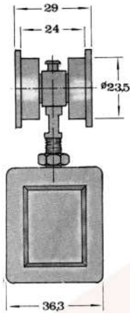
ROL 305 RETA Roldana com Rolamento e Guia DS 314
