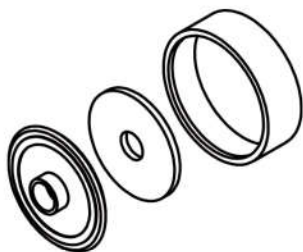
FIX 066 Fixador de Vidro Temperado Nylon Preto e Arruela de Aço Zincado
