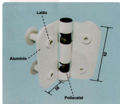
1756 Dobradiça Automática Dupla Granito/Madeira/Vidro Acabamento Branco ou Polido
