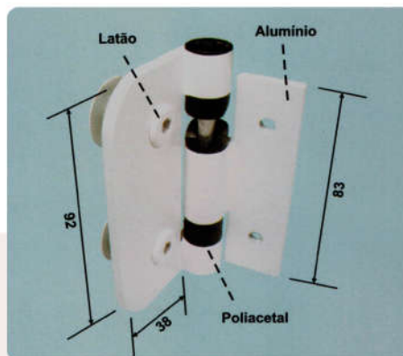
1755 Dobradiça Automática Granito/Alvenaria/Vidro Acabamento Branco ou Polido
