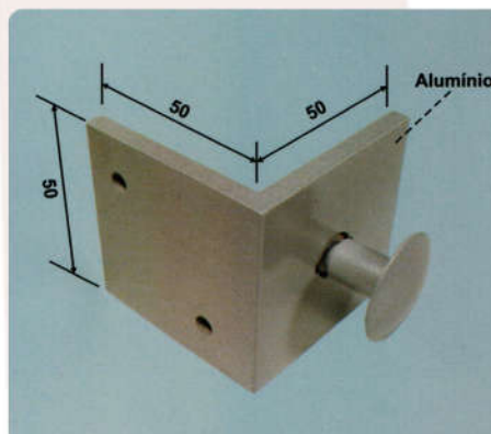
1760 Cantoneira Granito/Alvenaria Acabamento Branco ou Polido
