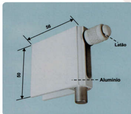
1800AS Trinco de Pressão para Janela de Correr Acabamento Branco ou Polido
