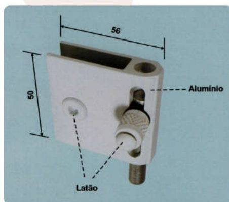
1800 Trinco para Janela de Correr Acabamento Branco ou Polido
