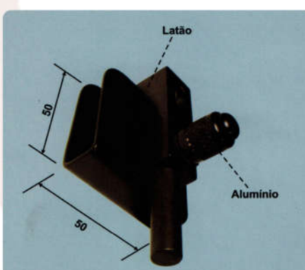
1800C Trinco de Pressão sem Núcleo Acabamento Branco ou Polido
