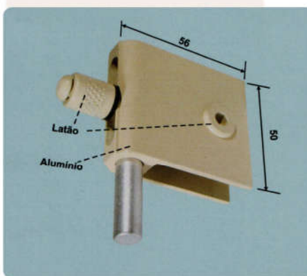
1800A Trinco para Janela de Correr Acabamento Branco ou Polido
