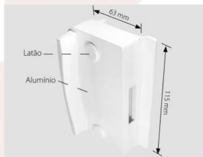
1511X VSM Contra Fechadura Porta de Correr Modelo 2 V/V Acabamento Branco ou Polido
