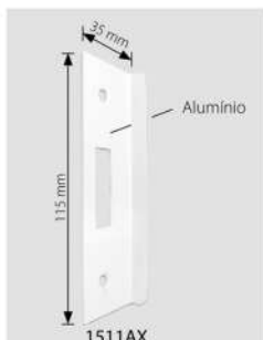
1511AX VSM Contra Fechadura Porta de Correr Modelo 2 V/A Acabamento Branco ou Polido
