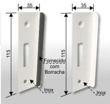
1511AX PACRE Contra Fechadura Porta de Correr V/A Acabamento Branco ou Polido
