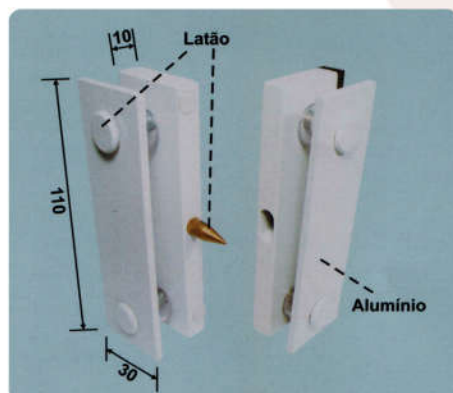
1710 Conjunto Mão-de-Amigo p/ Portas de Correr c/ 1030 Acabamento Branco ou Polido
