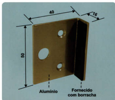
1400 Batedeira para Trinco Basculante Acabamento Branco ou Polido
