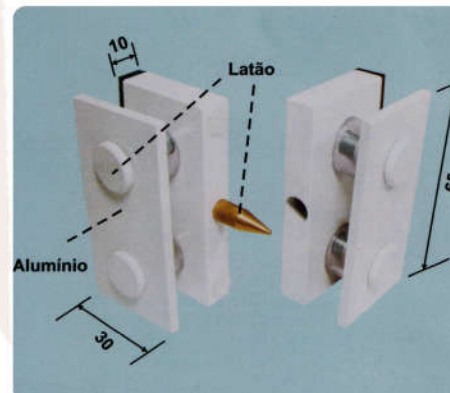
1710M Mini Conj. para Portas de Correr com 1030 Acabamento Branco ou Polido
