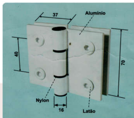
1131 Dobradiça Maxim-Ar V/V 40mm Acabamento Branco ou Polido
