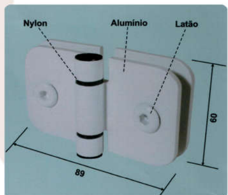
1137 Dobradiça Maxim-Ar 1 Furo V/V Acabamento Branco ou Polido
