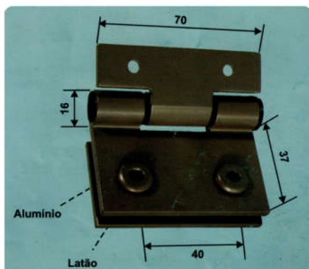
1132 Dobradiça Maxim-Ar V/A 40mm Acabamento Branco ou Polido
