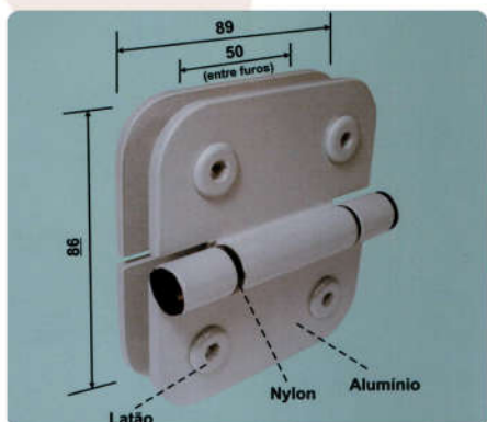
1134 Dobradiça Maxim-Ar V/V 50mm Acabamento Branco ou Polido
