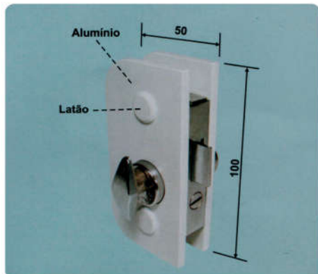
1520 BF Fechadura de Centro Bate-Fecha Acabamento Branco ou Polido
