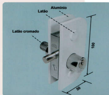
1501 Fechadura com Trinco Roleta Acabamento Branco ou Polido
