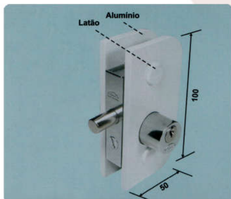
1502 Fechadura com Cilindro apenas de um lado Acabamento Branco ou Polido
