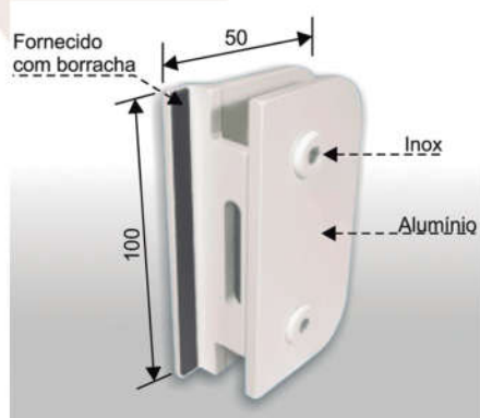
1531BF Batedeira V/V com Aba para 1520BF Acabamento Branco ou Polido
