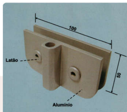
1519A Contra-Trinco sem Núcleo para 1519 Acabamento Branco, Polido
