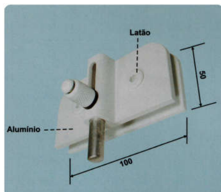
1519 Trinco Inferior sem Núcleo 50x100mm Acabamento Branco, Polido
