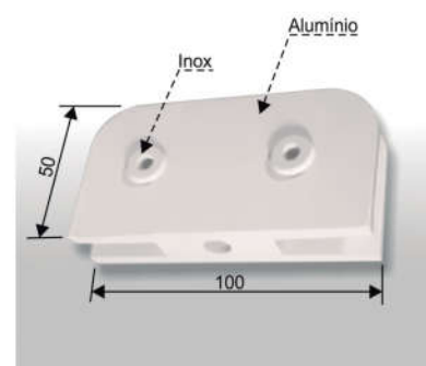
1231 Dobradiça Bucha Basculante 50x100 Acabamento Branco ou Polido
