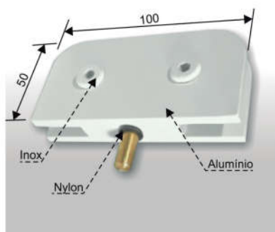
1130 Dobradiça Pino Basculante 50x100 Acabamento Branco ou Polido
