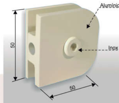
1230 Dobradiça Bucha Basculante 50x50 Acabamento Branco ou Polido
