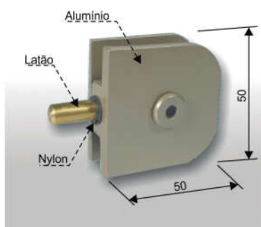
1123 Dobradiça Pino Basculante 50x50 Acabamento Branco ou Polido
